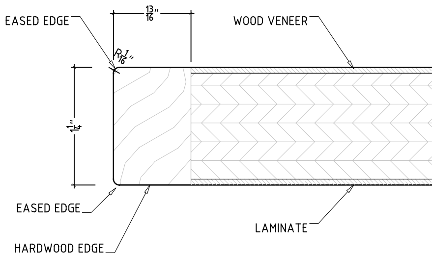
4 EDGE DETAIL SCALE: FULL SCALE
