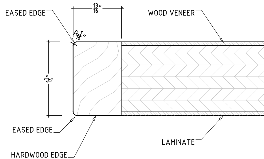
4 EDGE DETAIL SCALE: FULL SCALE
