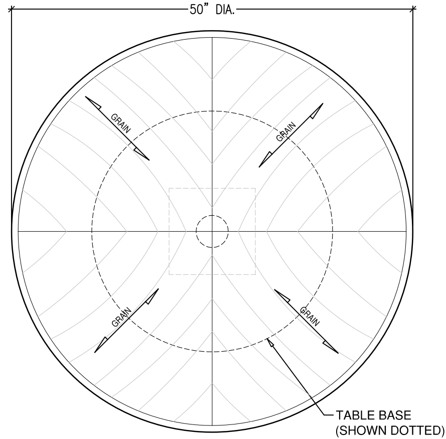
TOP VIEW 1 PLAN SCALE: 1" = 1'-0"
