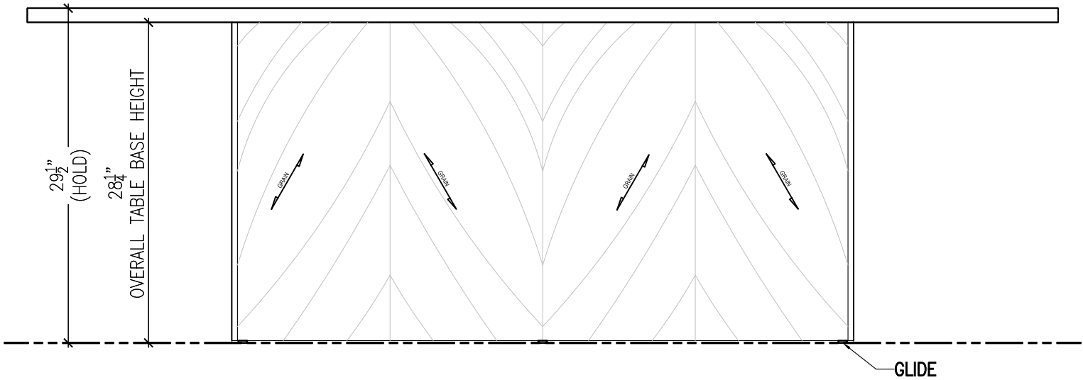
2 ELEVATION SCALE: 1" = 1'-0"
