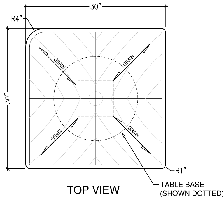
1 PLAN SCALE: 1" = 1' - 0"
