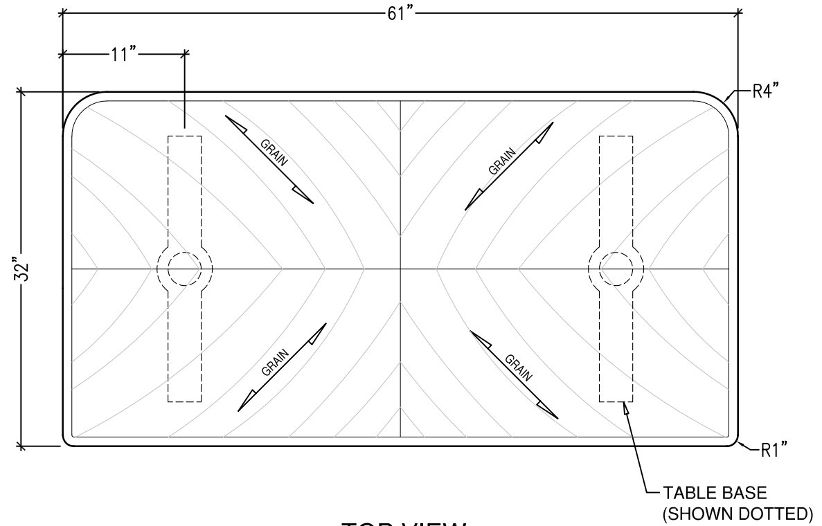
TOP VIEW 1 PLAN SCALE: 1" = 1' - 0"
