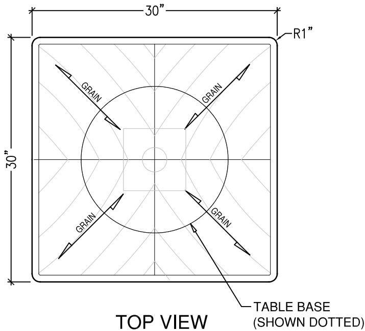
1 PLAN SCALE: 1" = 1' - 0"
