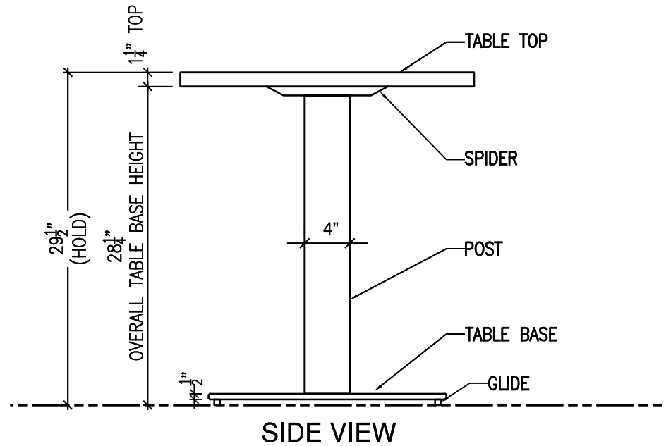
3 ELEVATION SCALE: 1" = 1'-0"
