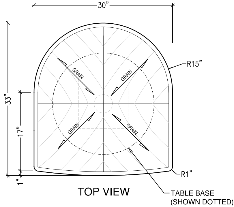
1 PLAN SCALE: 1" = 1' - 0"
