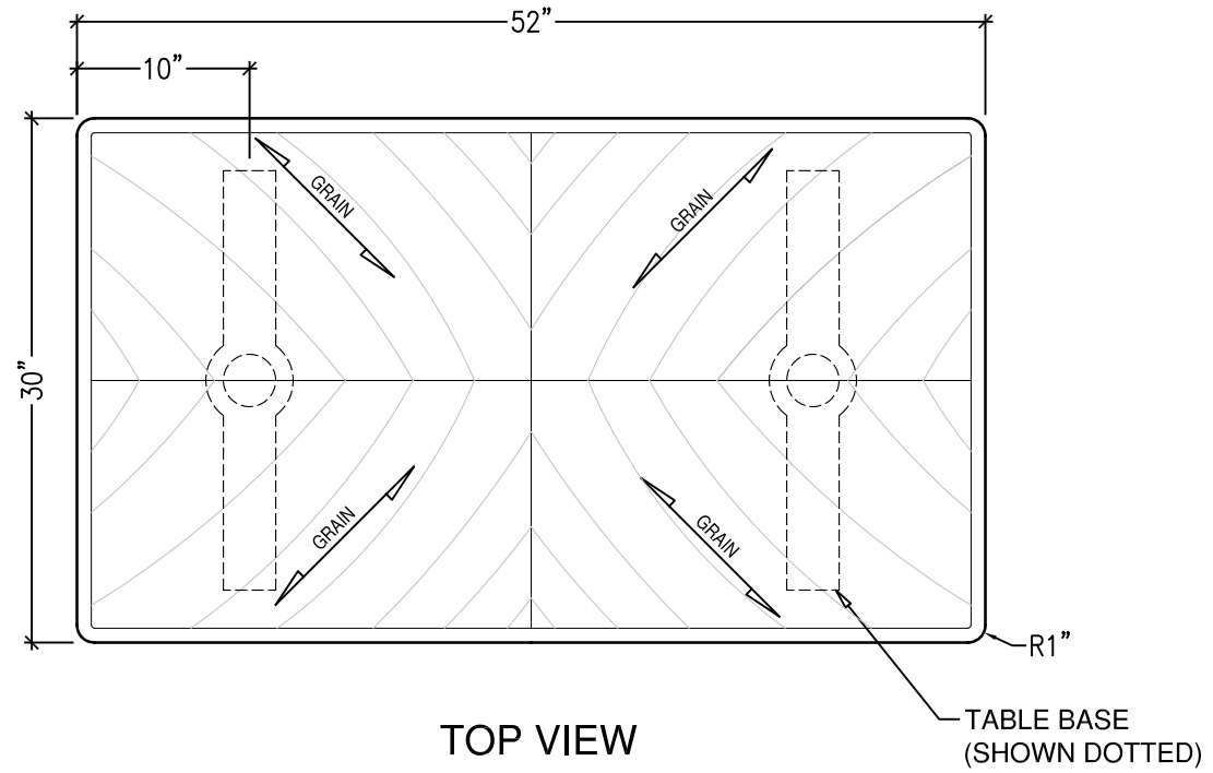
1 PLAN SCALE: 1" = 1' - 0"
