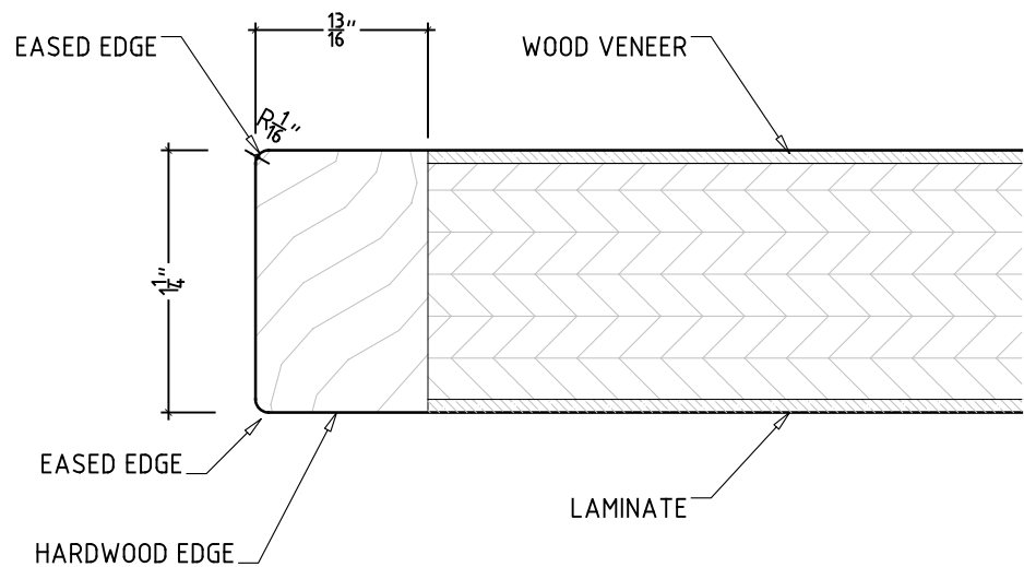
4 EDGE DETAIL SCALE: FULL SCALE
